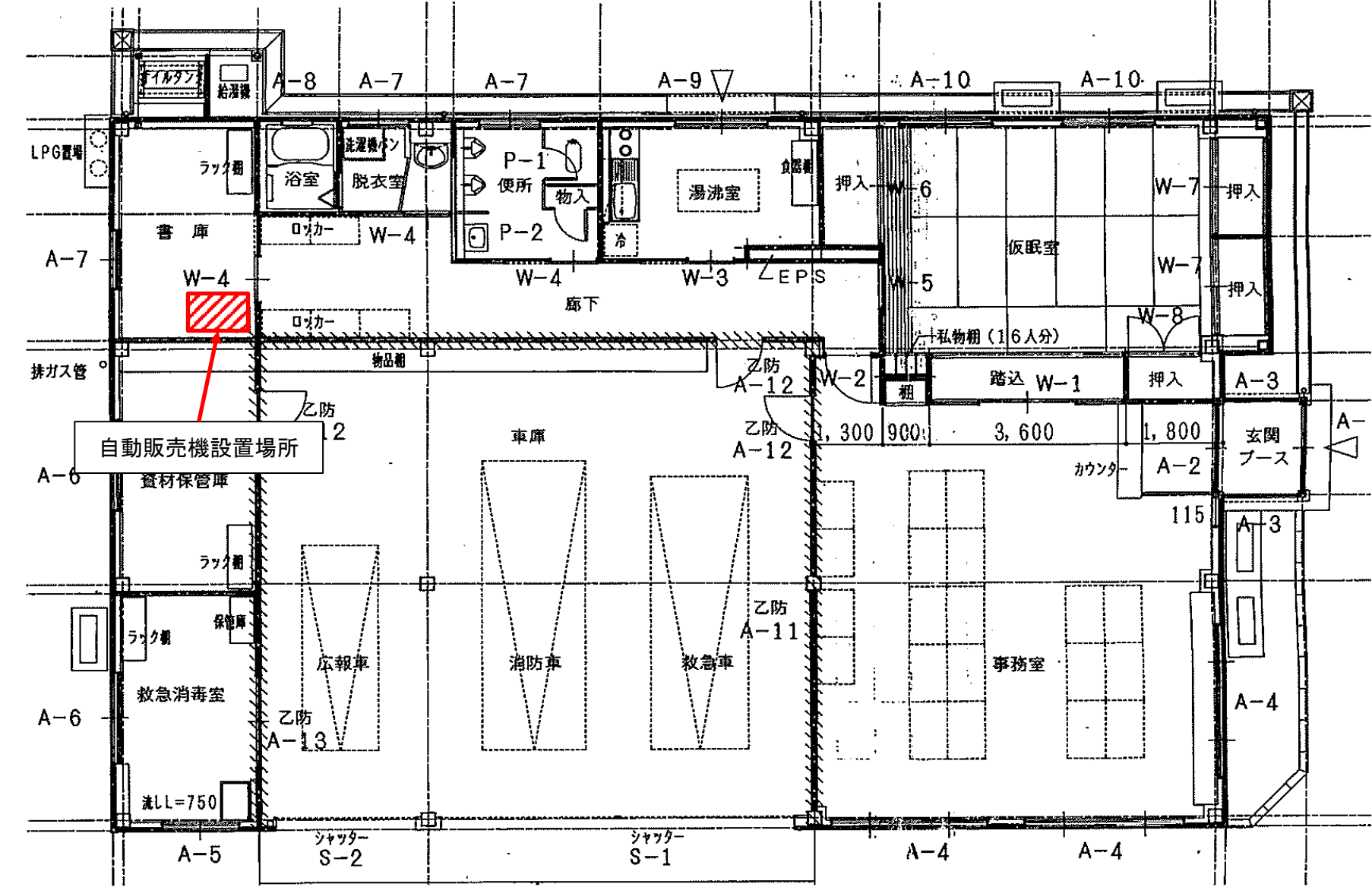
物件番号 5 村上市消防署山北分署1階平面図
