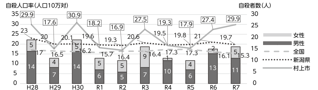
図1 自殺の現状
