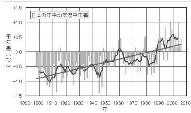
図 2-2-7 日本における年平均気温の経年変化(1898～2006年)
