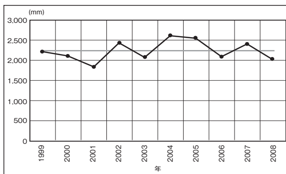
図2-2-3 村上市の過去10年間（1999～2008年）の月降水量 （資料：気象庁電子資料室・村上観測所）
