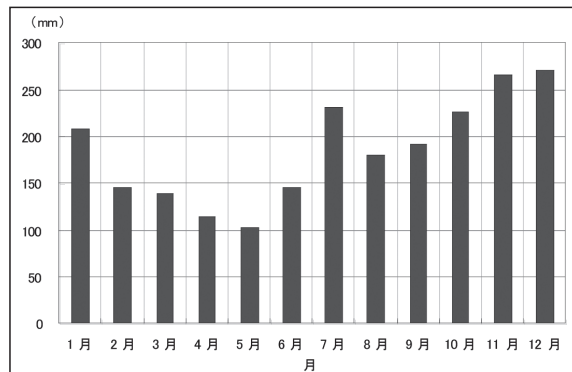
図2-2-2 村上市の過去10年間(1999～2008年)の月降水量 (資料:気象庁電子資料室・村上観測所)
