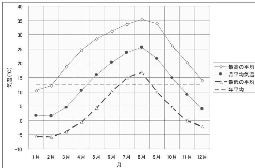
図2-2-1 村上市の過去10年間(1999～2008年)の月平均気温
