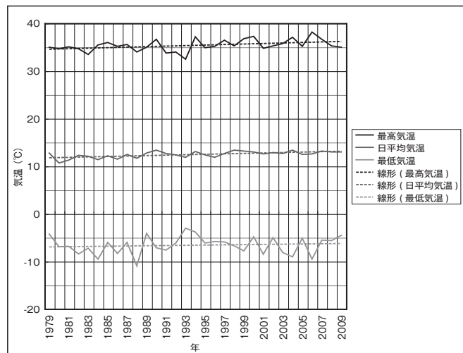
図 2-2-8 村上市の過去30年間の平均・最高・最低気温の推移(資料：気象庁 2009)
