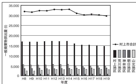
図 2-2-5 村上市の一般廃棄物の排出量の推移
