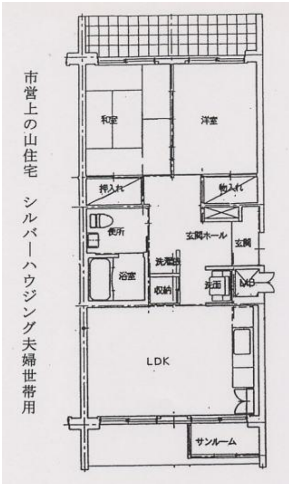
【間取図】
